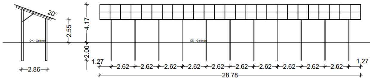
Abbildung 9: Schnittdarstellung Solarmodule, o. M. (Verfasser: maxsolar)
