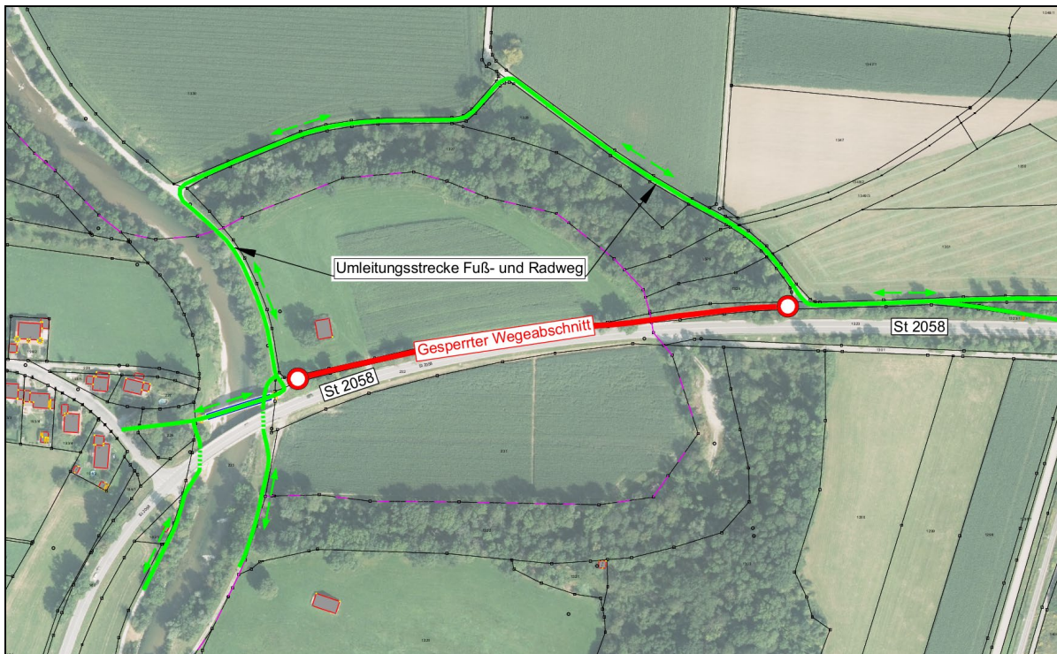
Lageplan Sperrung/Umleitung Radfahrer und Fußgänger
